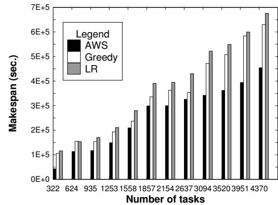
Fig. 3. Makespan.
